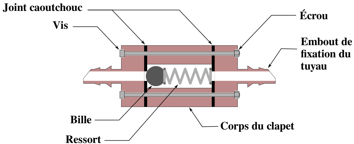
Clapet à bille
